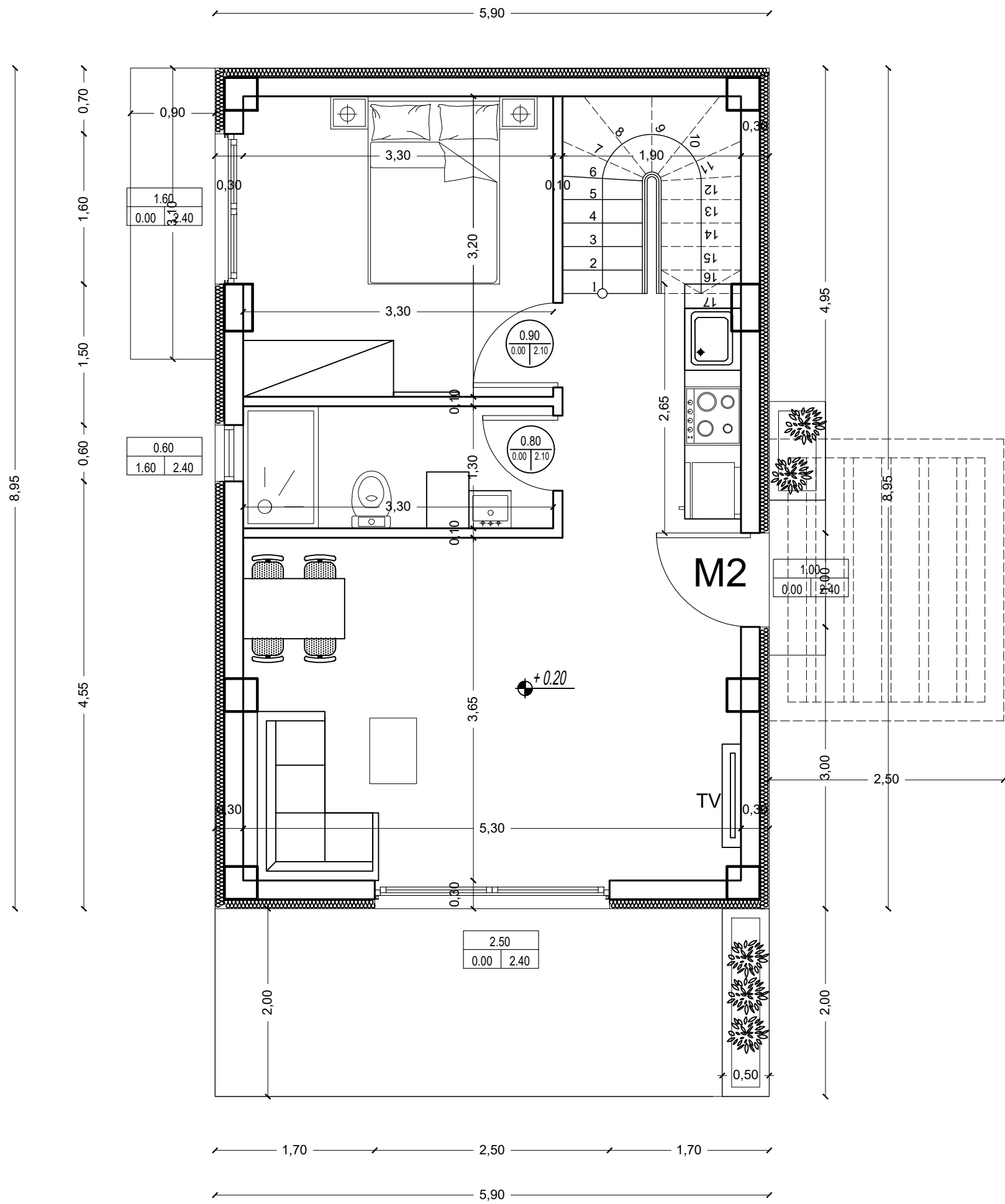
ΚΑΤΟΨΗ ΙΣΟΓΕΙΟΥ M2
